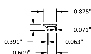
19 LOCK BAR BASE 6063-T5
