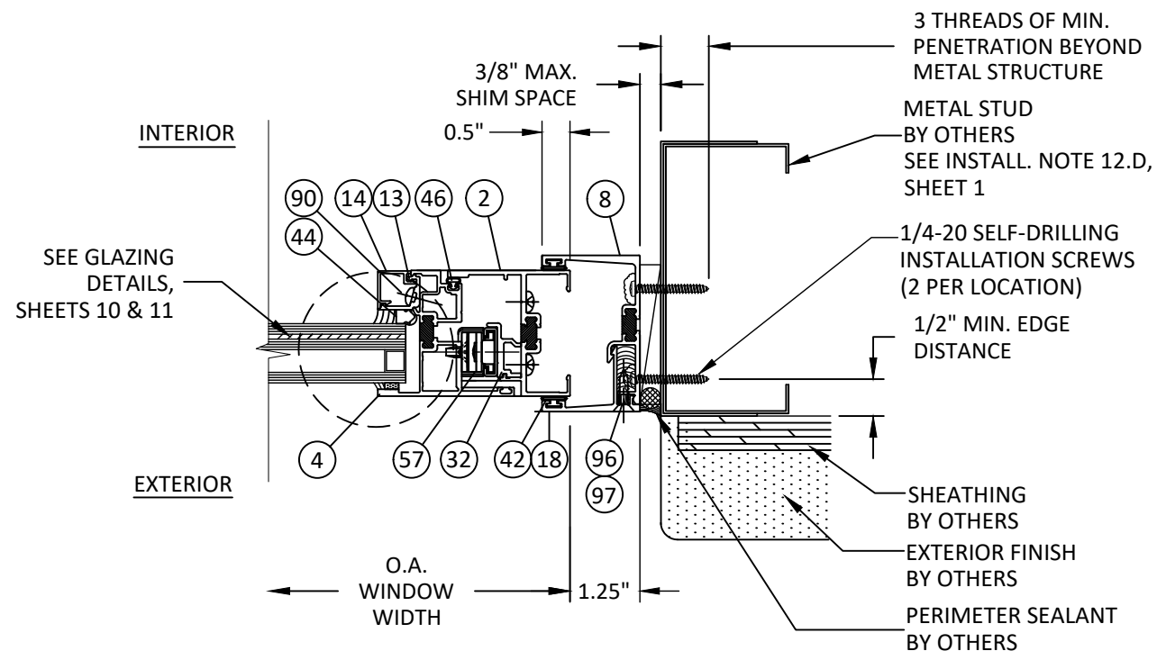
C 4 HORIZONTAL SECTION VENT JAMB - METAL STUD FRAME EXT. SET RECEPTOR - TYP.
